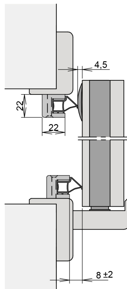
Horizontalschnitt
